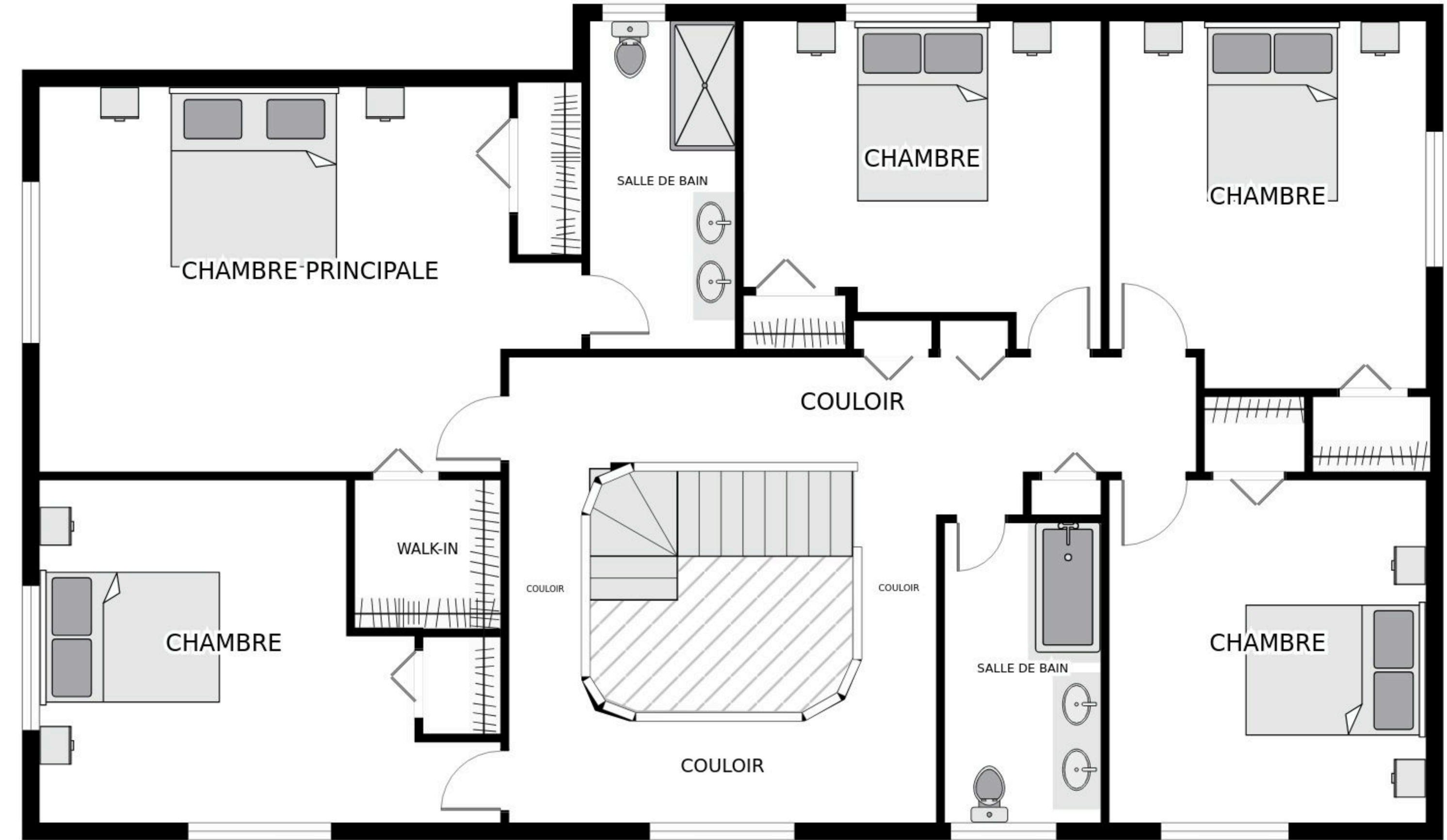
DEUXIÈME ÉTAGE
